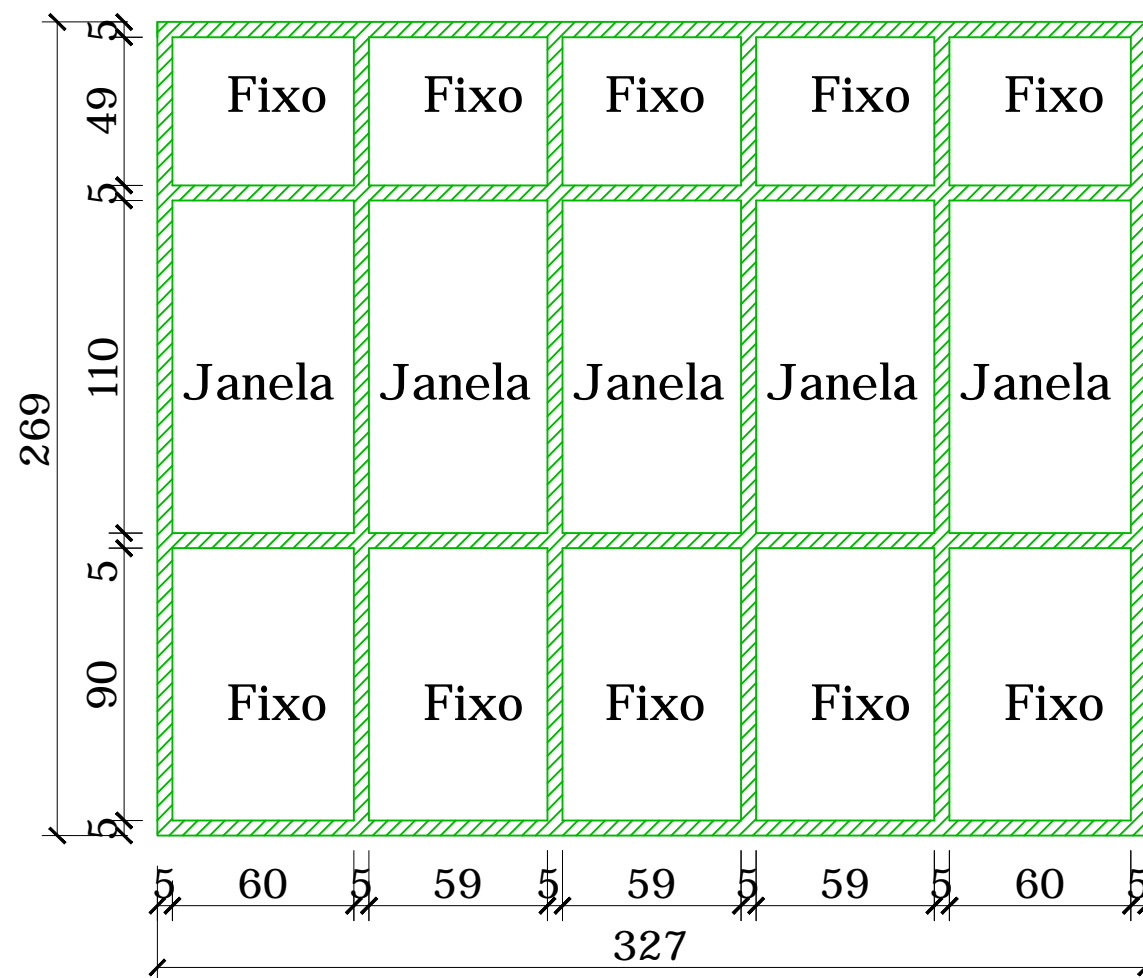
Dimensões da Estutura 06 Tubos de Aço 50x30x2 mm
