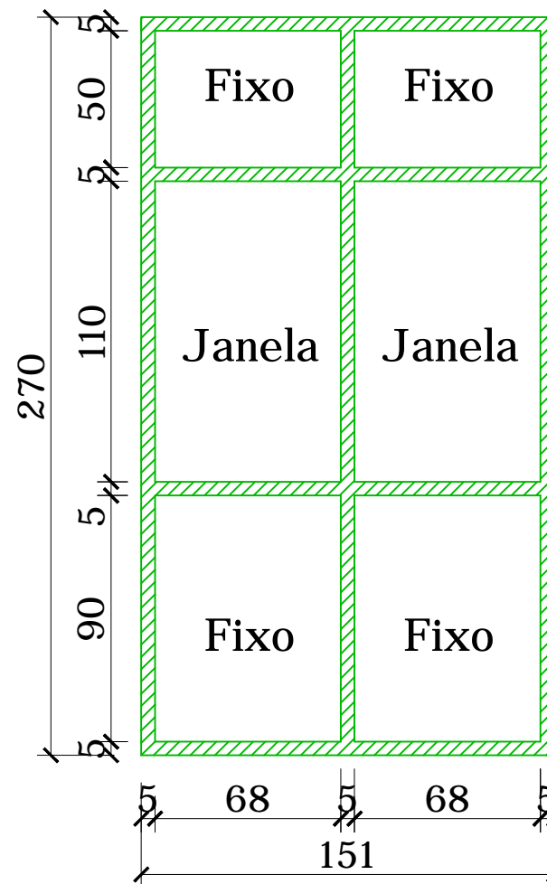
Dimensões da Estutura 07 Tubos de Aço 50x30x2 mm
