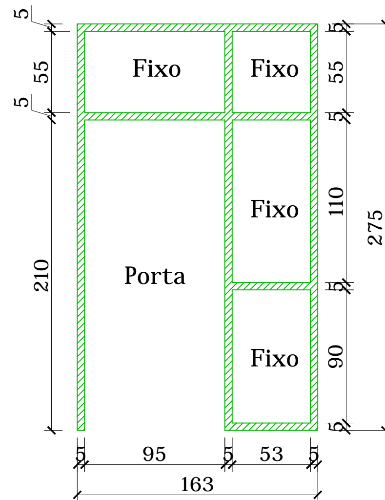
Dimensões da Estutura 08 Tubos de Aço 50x30x2 mm
